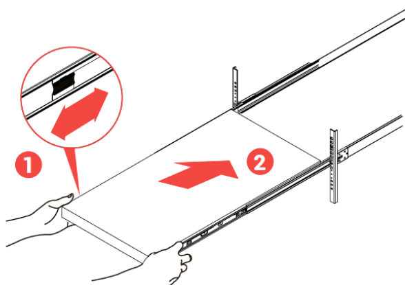
Рисунок 30 – Установка изделия в стойку
