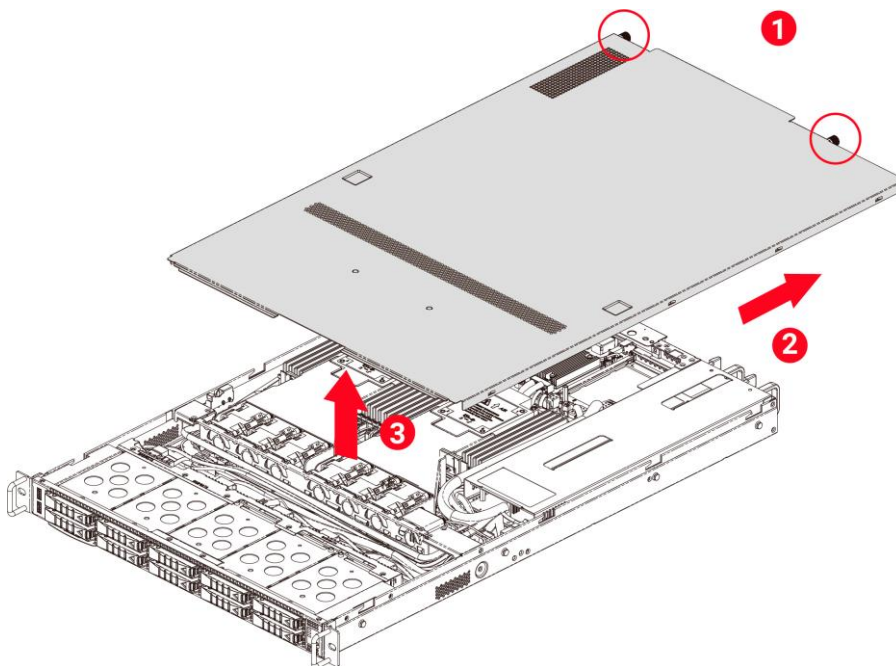
Рисунок 17 – Монтаж верхней крышки сервера
