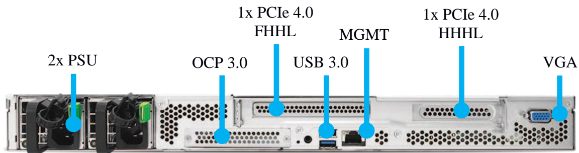
Рисунок 4 – Функциональные элементы, расположенные на задней панели корпуса изделия
