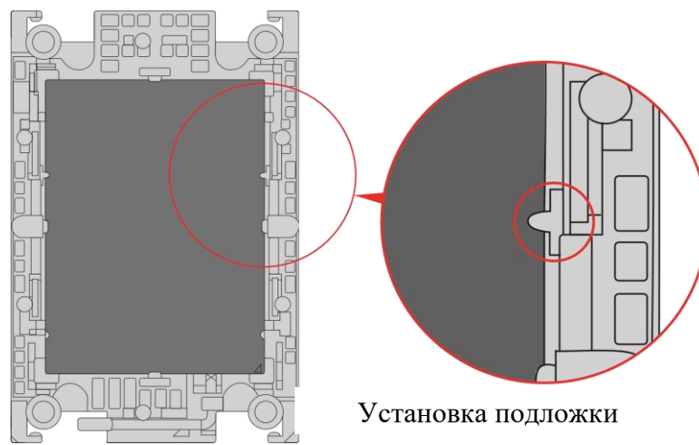
Рисунок 9 – Установка подложки
