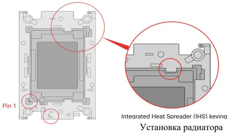
Рисунок 8 – Установка радиатора
