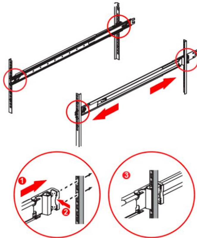
Рисунок 29 – Установка внешних направляющих
