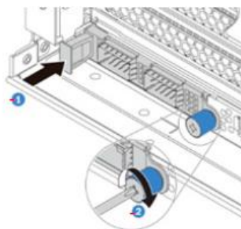
Рисунок 25 – Установка Ethernet – адаптера OCP 3.0
