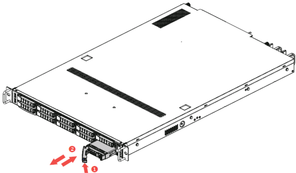
Рисунок 20 – Снятие каретки для накопителей 2,5”
