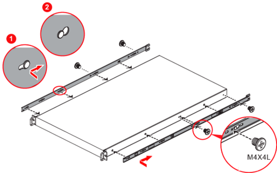
Рисунок 28 – Установка внутренних направляющих
