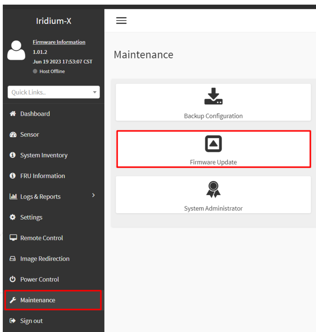
Рисунок 1 – Вкладка Maintenance
