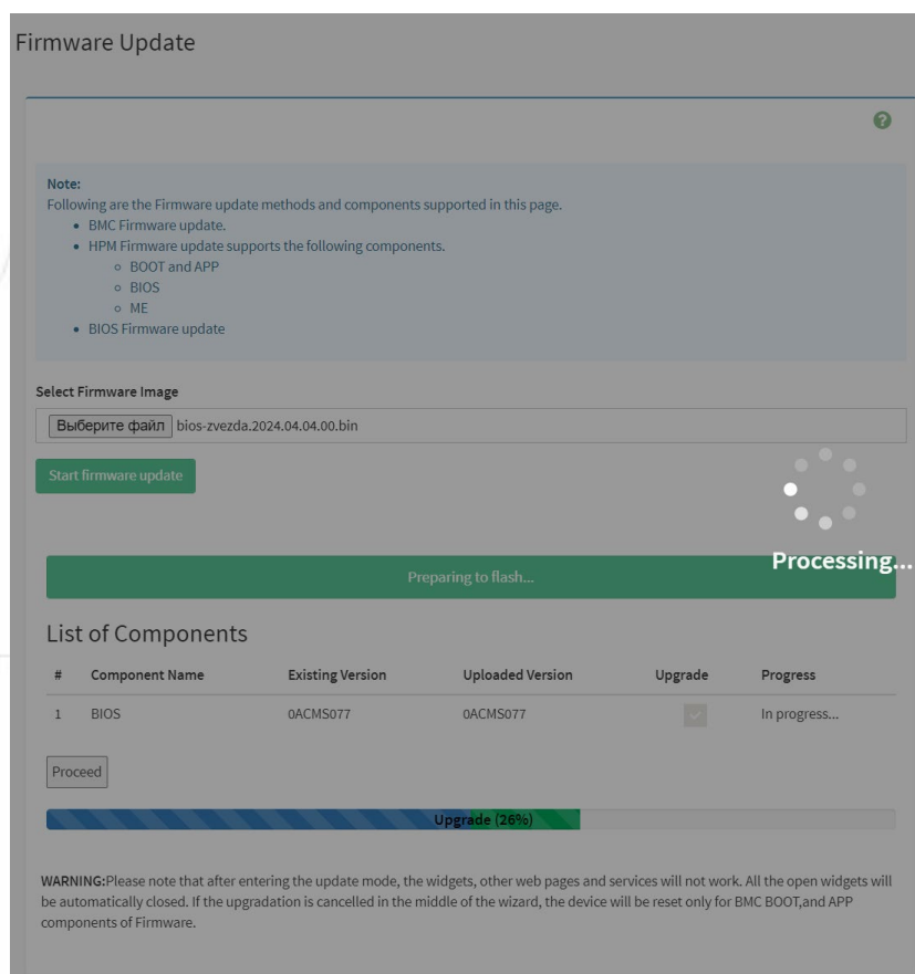
Рисунок 5 – Обновлений системы
