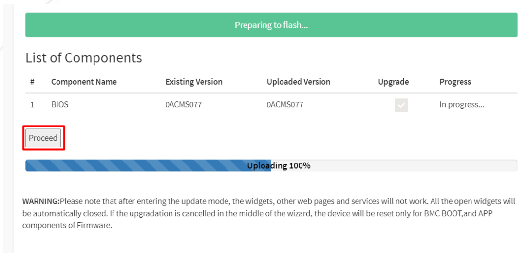
Рисунок 4 – Загрузка файла
